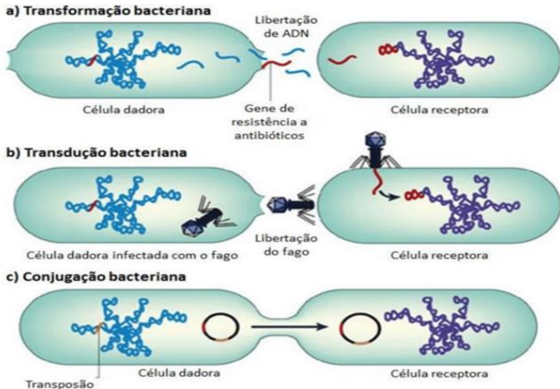
Figura 1. Esquematização dos mecanismos de resistência bacteriana adquirida por transferência horizontal de genes: a) transformação, b) transdução c) conjugação. Adaptado de (TEIXEIRA; FIGUEIREDO; FRANÇA, 2019).
